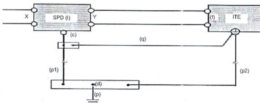
图 J.2.4-2 将多接线端子电涌保护器的有效电压保护水平
