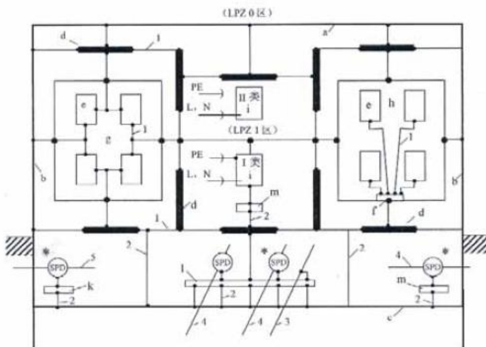
图 6.3.3 接地、等电位连接和接地系统的构成
