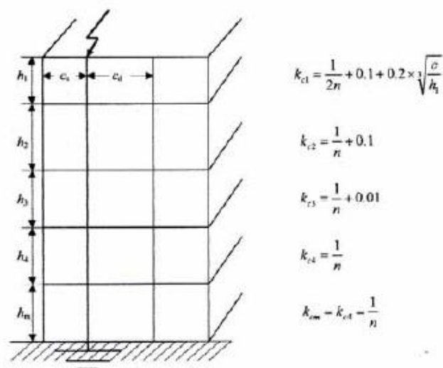
图 E.0.2 分流系数 k_c ( 2 )
