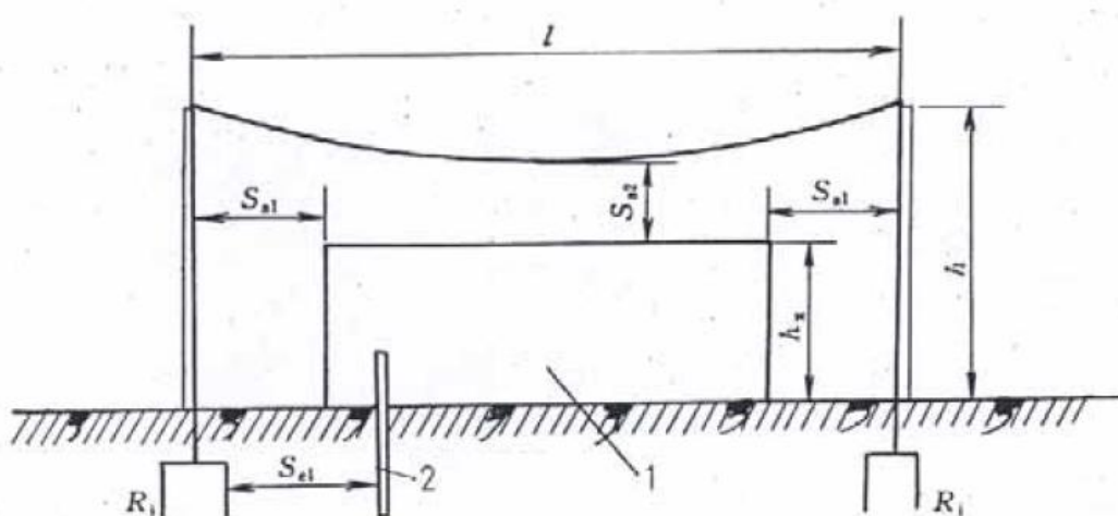
图 4.2.1 防雷装置至被保护物的间隔距离
