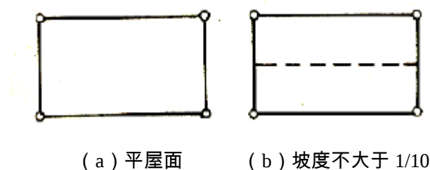
图 B.0.1 建筑物易受雷击的部位（一）
