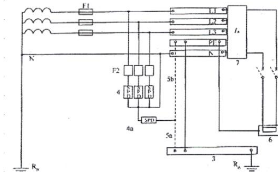
图 J.1.2-2 TT 系统电涌保护器安装在进户处 RCD 的电源侧
