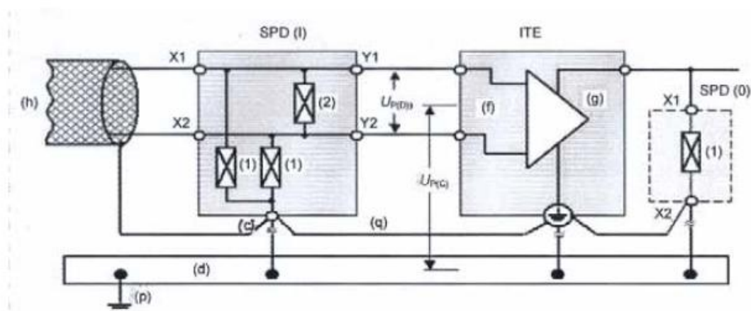
图 J.2.3-1 防需要保护的电子设备 (ITE)的供电电压输入端
