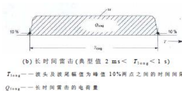
图 F.0.1-2 雷击参数定义
