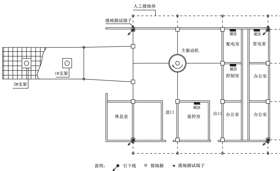
图 B.2 站房防雷接地平面图
